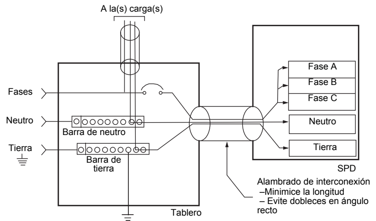
Figura 2: Alambrado del SPD para las configuraciones en delta con extremo alto y en estrella
