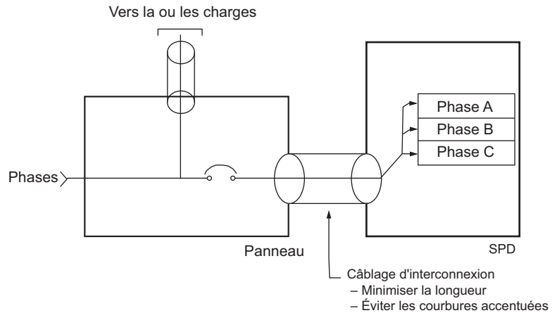
Figure 3: Câblage du SPD pour les configurations en triangle
